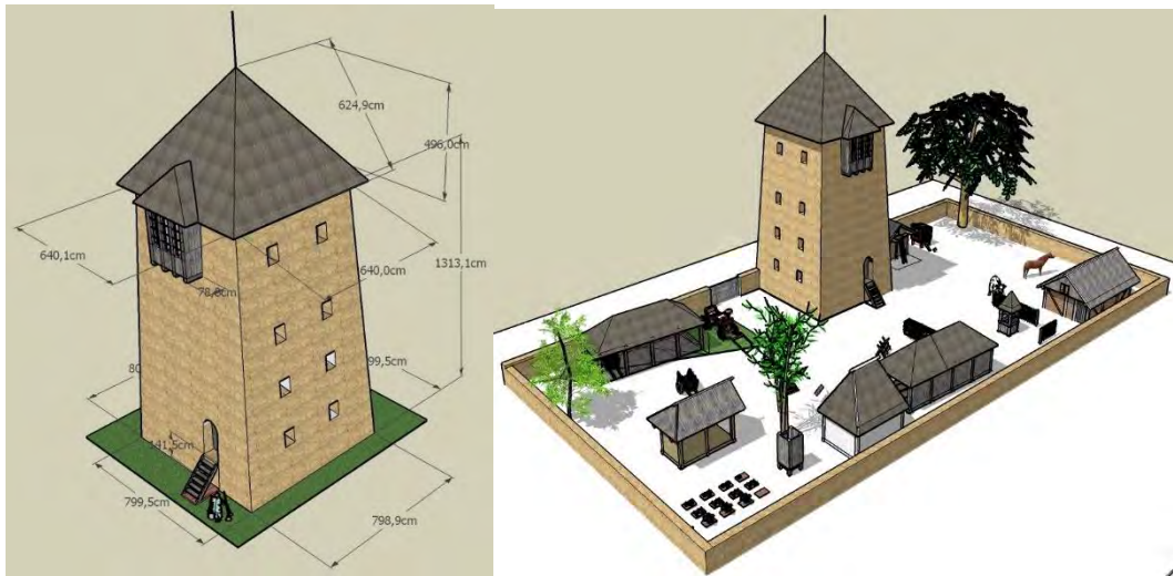
Sl. 8. i 9: Perspektivni izgled kule i avlije; perspektivni izgled i veličina kule
